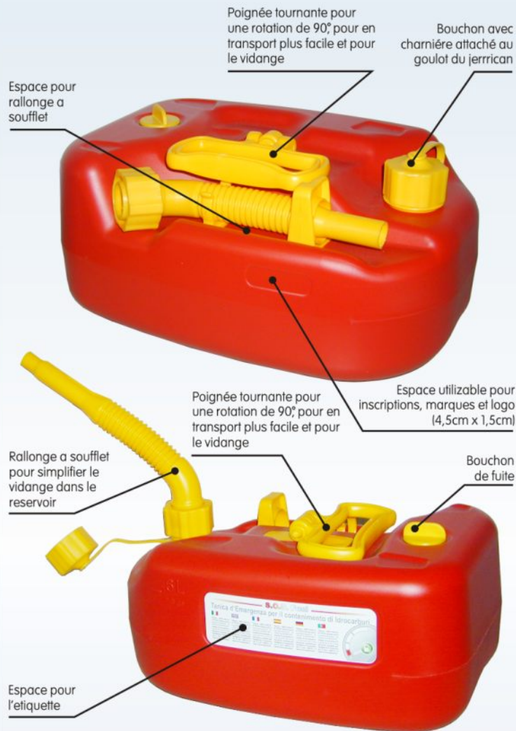
Avec la rallonge a soufflet inclinée on peut remplir tous les modèles de réservoirs (voiture et moto mais équipement de jardin aussi)
