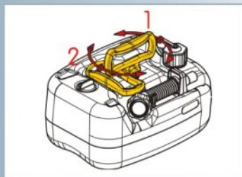
Dessin de la Poignée électrique pour expliquer la rotation: Pos.1 pour un transport plus facile; Pos. 2 pour un vidange plus facile
